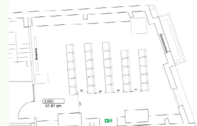
Reihenbestuhlung
