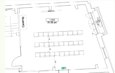
Reihenbestuhlung
